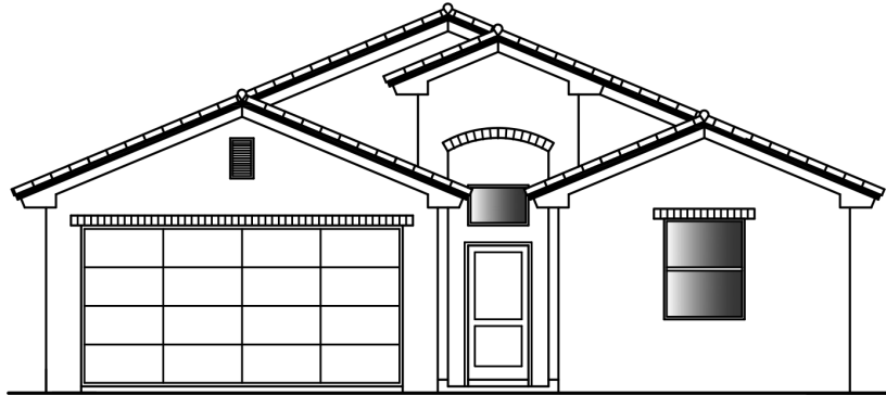
ELEVATION A
